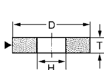
Suora hiomalaikka (Tyyppi 1)
