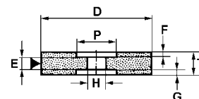
Kaksoisporaus (Tyyppi 7)
