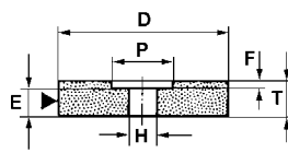
Yksinkertainen poraus (Tyyppi 5)
